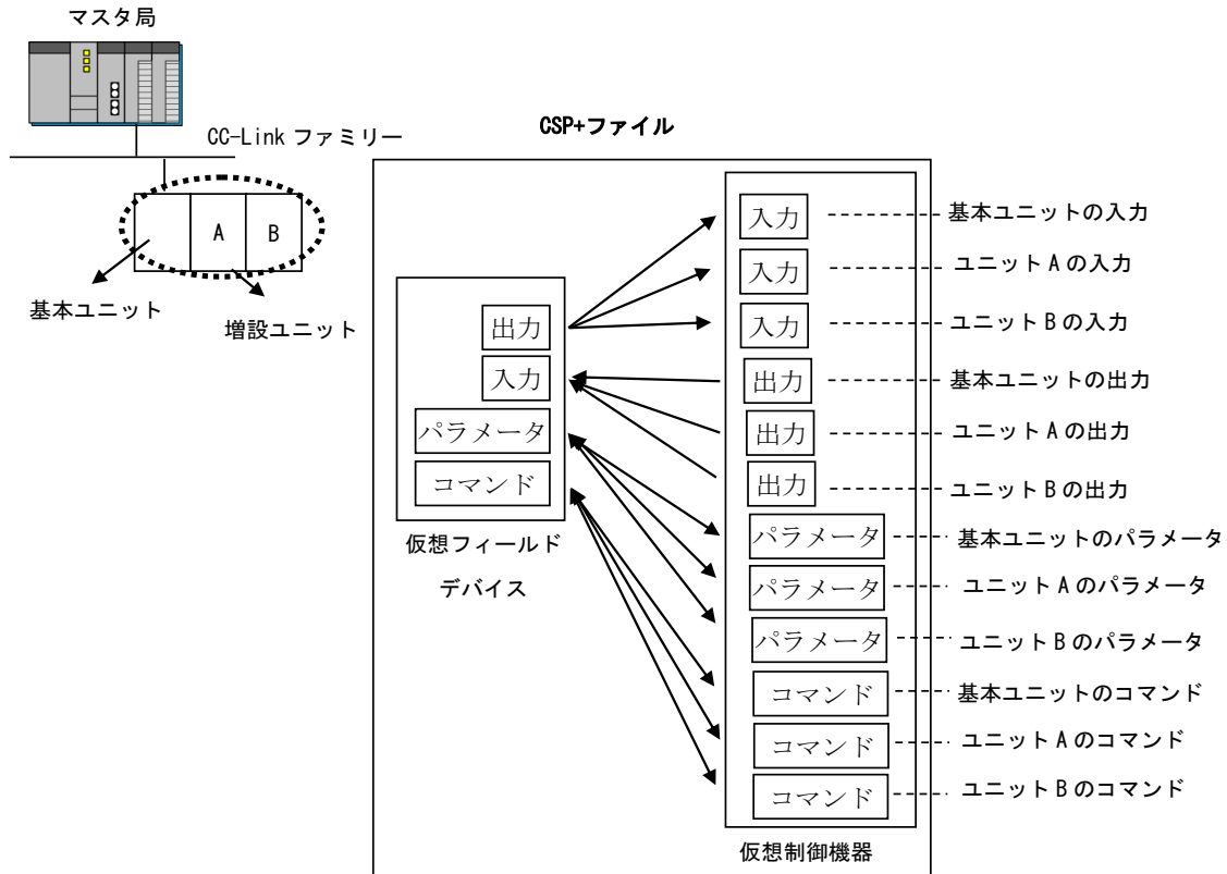
図 3-12 増設ユニットを含む構成で記述する場合のユニットのモデル(基本ユニットと増設ユニットの仮想制御機器をまとめて記述する場合)
