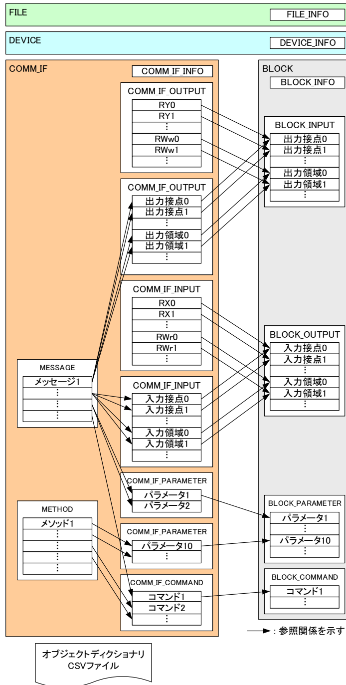
図 4-15 CC-Link IE TSN接続ユニット用CSP+ファイルの一般形モデル
