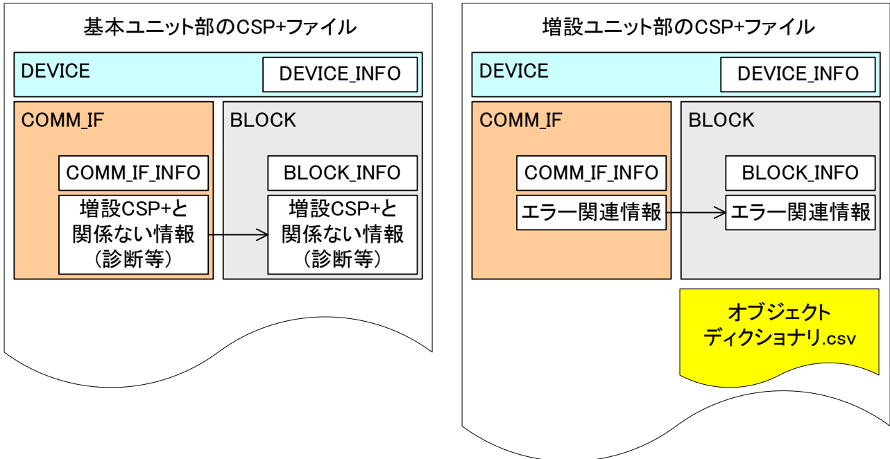
図 4-18 基本増設一体型ユニットのCSP+ファイルの一般型モデル
