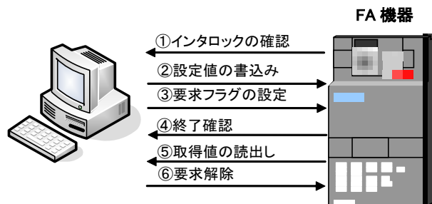
図 5-20 手順を用いた通信サービスの流れ
