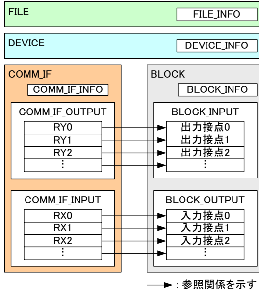
図 4-10 CC-Link IEフィールドネットワーク接続リモートI/O用CSP+ファイルのモデル
