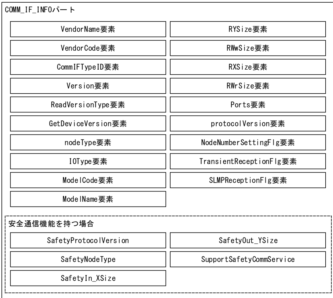
図 5-11 COMM_IF_INFOパートの構造 (CC-Link IEフィールドネットワークの場合)
