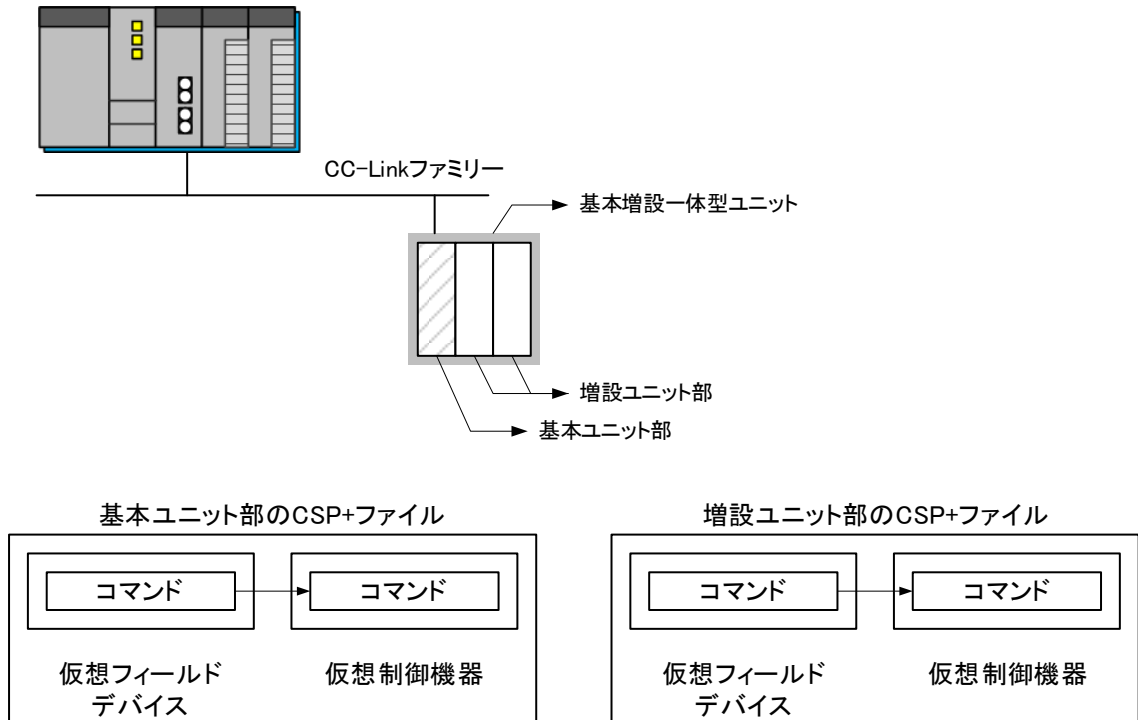
図 3-15 基本増設一体型ユニットのモデル
