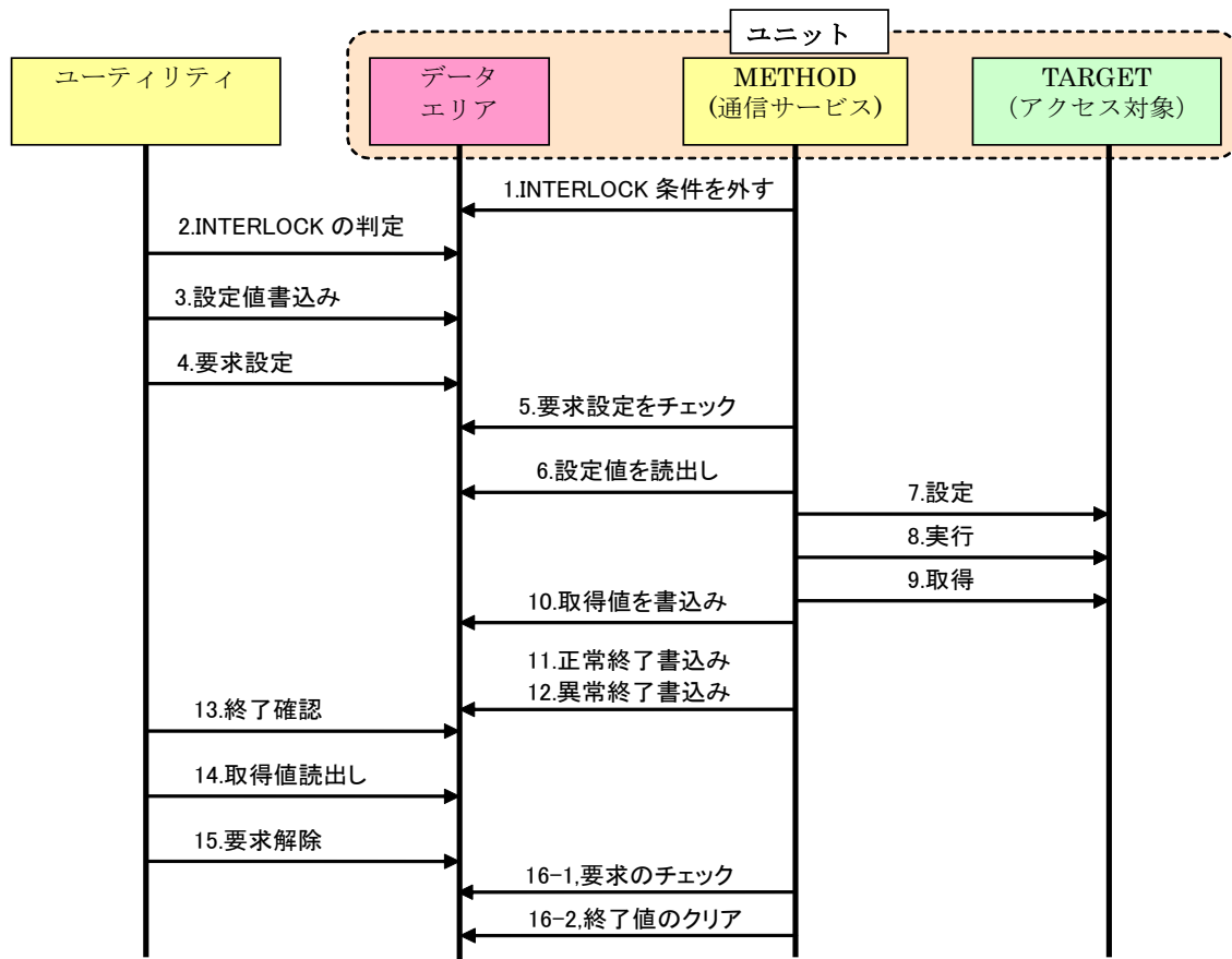
図 5-22 METHODのシーケンス
