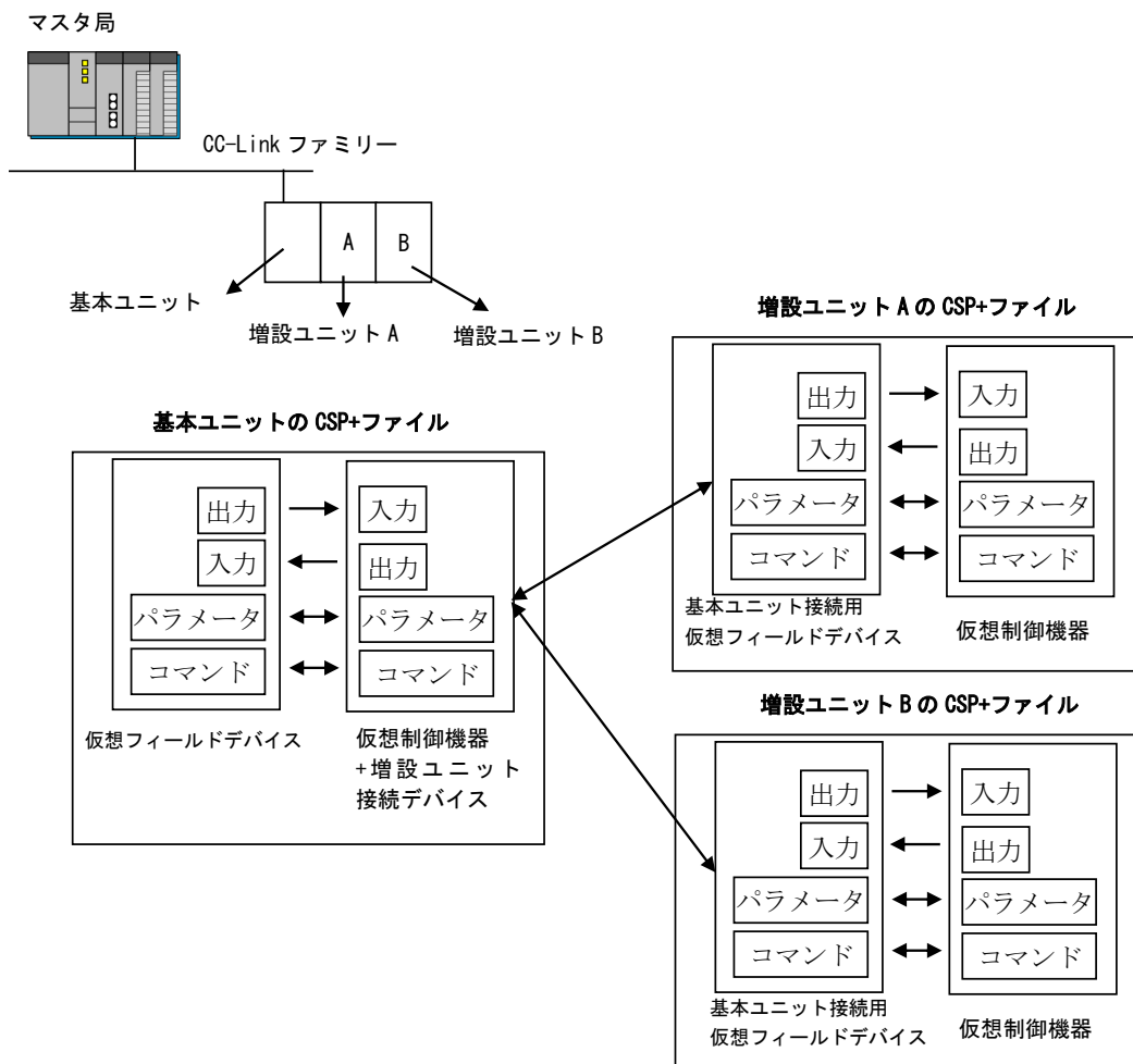
図 3-13 基本ユニットと増設ユニットのそれぞれで CSP+ファイルを作成する場合のモデル
