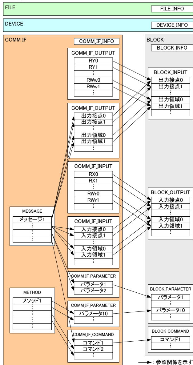
図4-11 CC-Link IEフィールドネットワーク接続リモートデバイス局、インテリジェントデバイス局、ローカル局用CSP+ファイルのモデル
