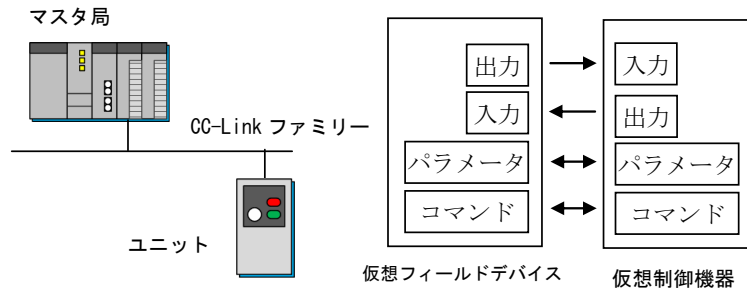
図 3-8 単一のネットワークに接続するユニットのモデル
