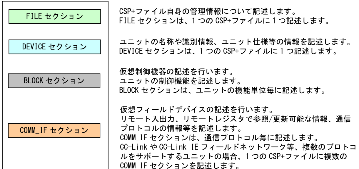
図 4-2 GSP+ファイルの構造
