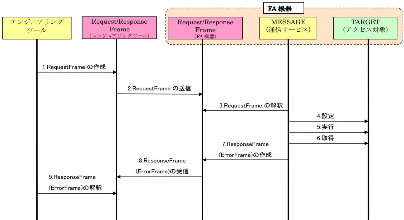
図 5-25 MESSAGEの呼び出しと動作シーケンス
