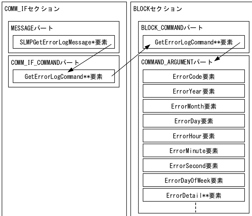
図 5-42 エラー履歴情報取得を記述する場合の構造イメージ(エラー情報をユニット本体側で管理する場合)
