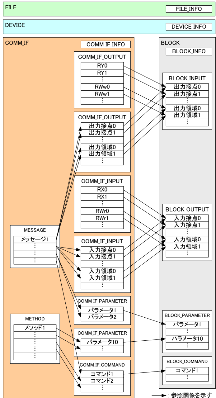
図 4-9 CC-Link IEフィールドネットワーク接続ユニット用GSP+ファイルの一般形モデル
