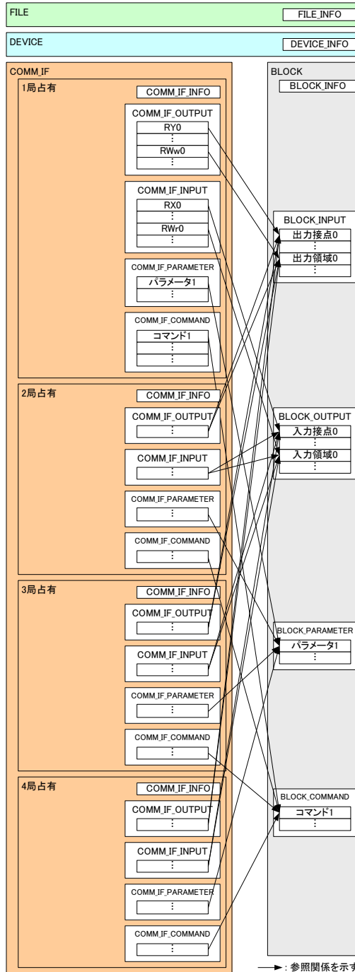
図 4-14 Ethernet接続ユニットでの複数のCOMM_IFセクション記述
