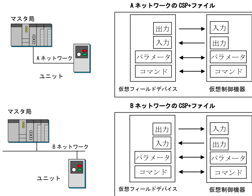
図 3-9 複数のネットワークを切り替えて使用するユニットのモデル
