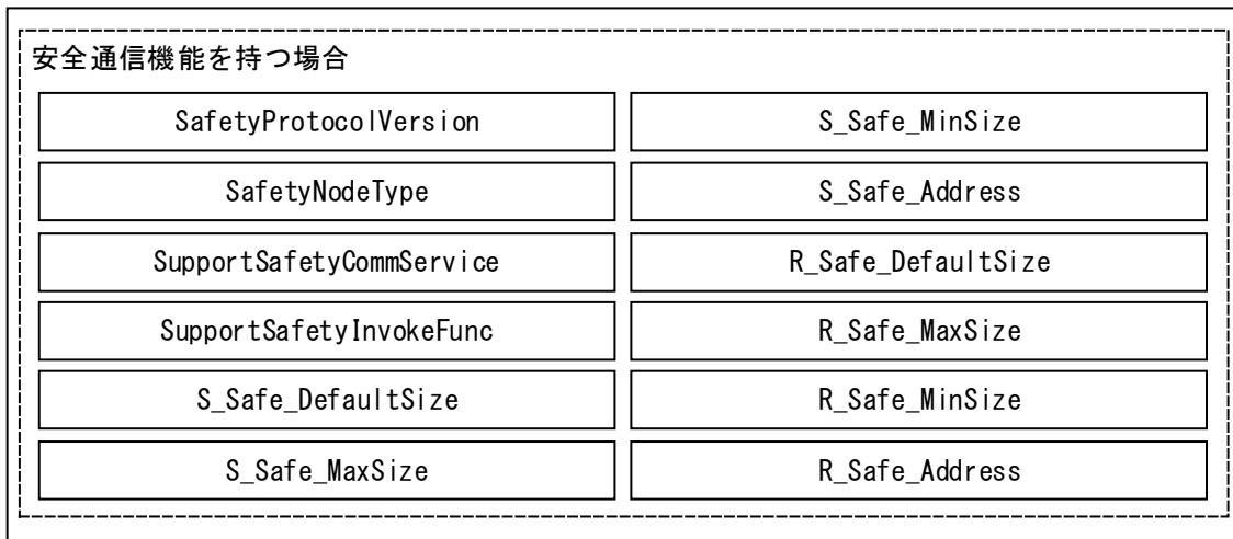
図 5-14 CC-Link IE TSN安全通信機能を持つ場合の詳細構造
