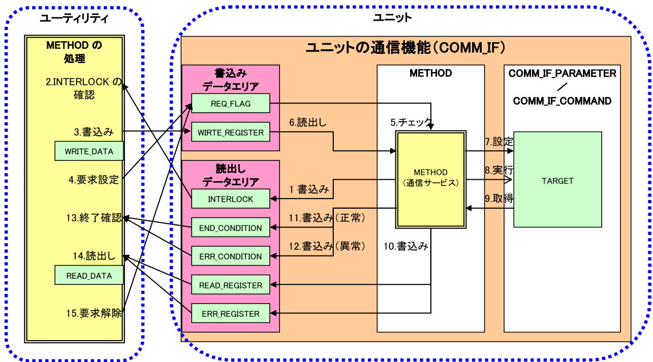
図 5-21 METHODで記述された通信サービスの動作
