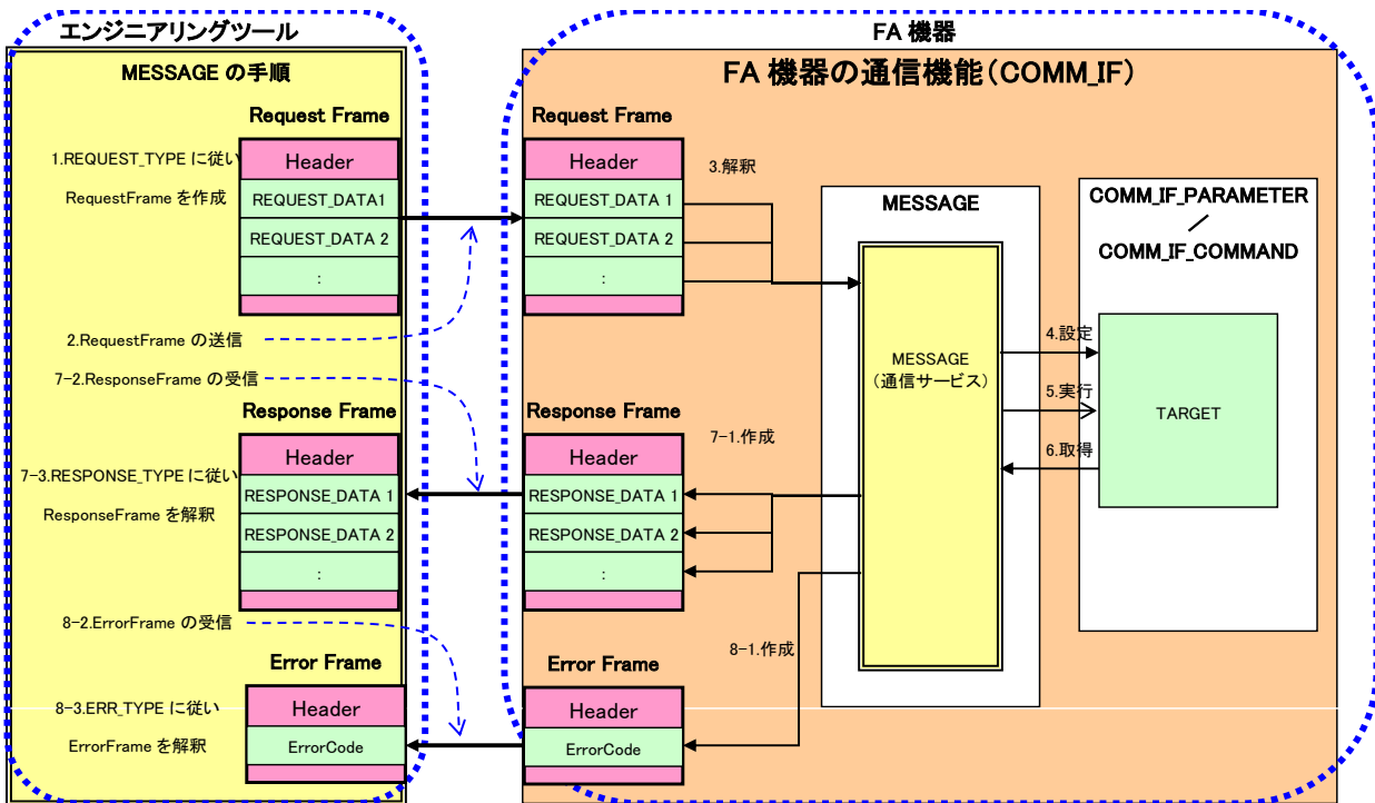
図 5-24 MESSAGEで記述された通信サービスの動作
