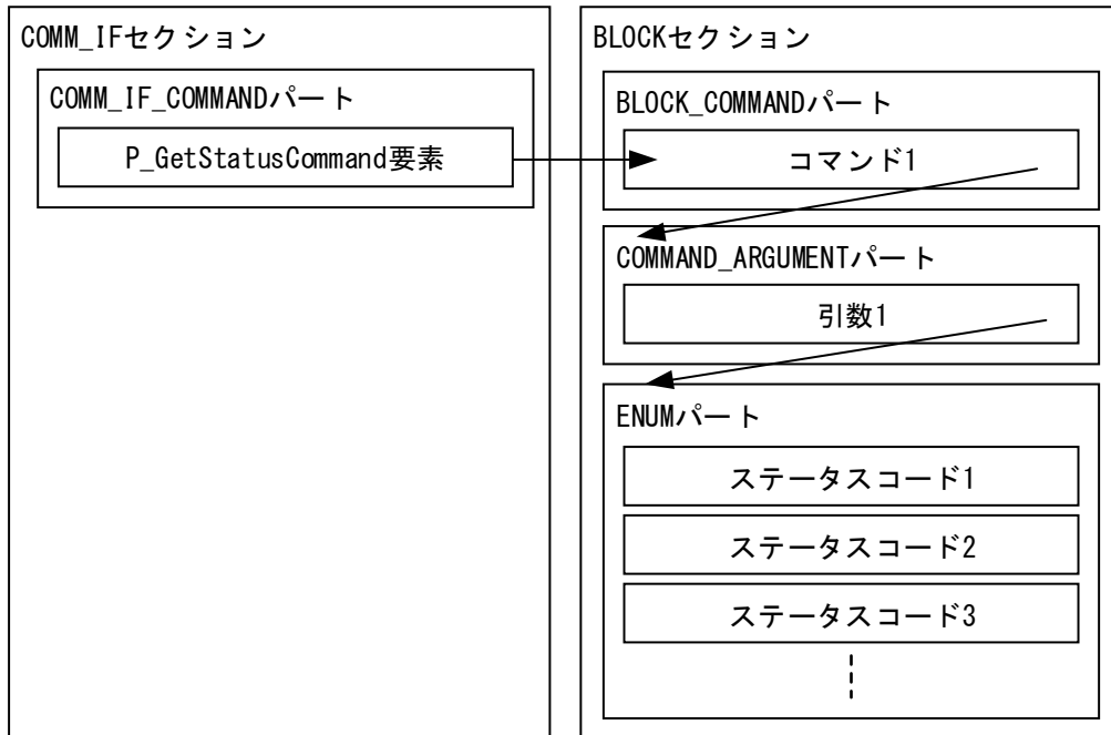
図 5-53 ステータス情報の取得を記述する場合の構造イメージ
