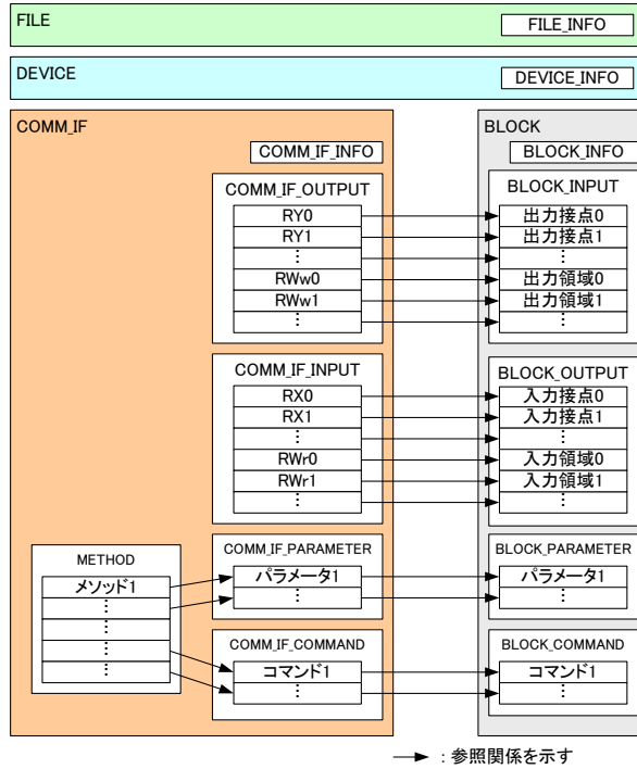
図 4-5 CC-Link接続ユニット用CSP+ファイルの一般形モデル
