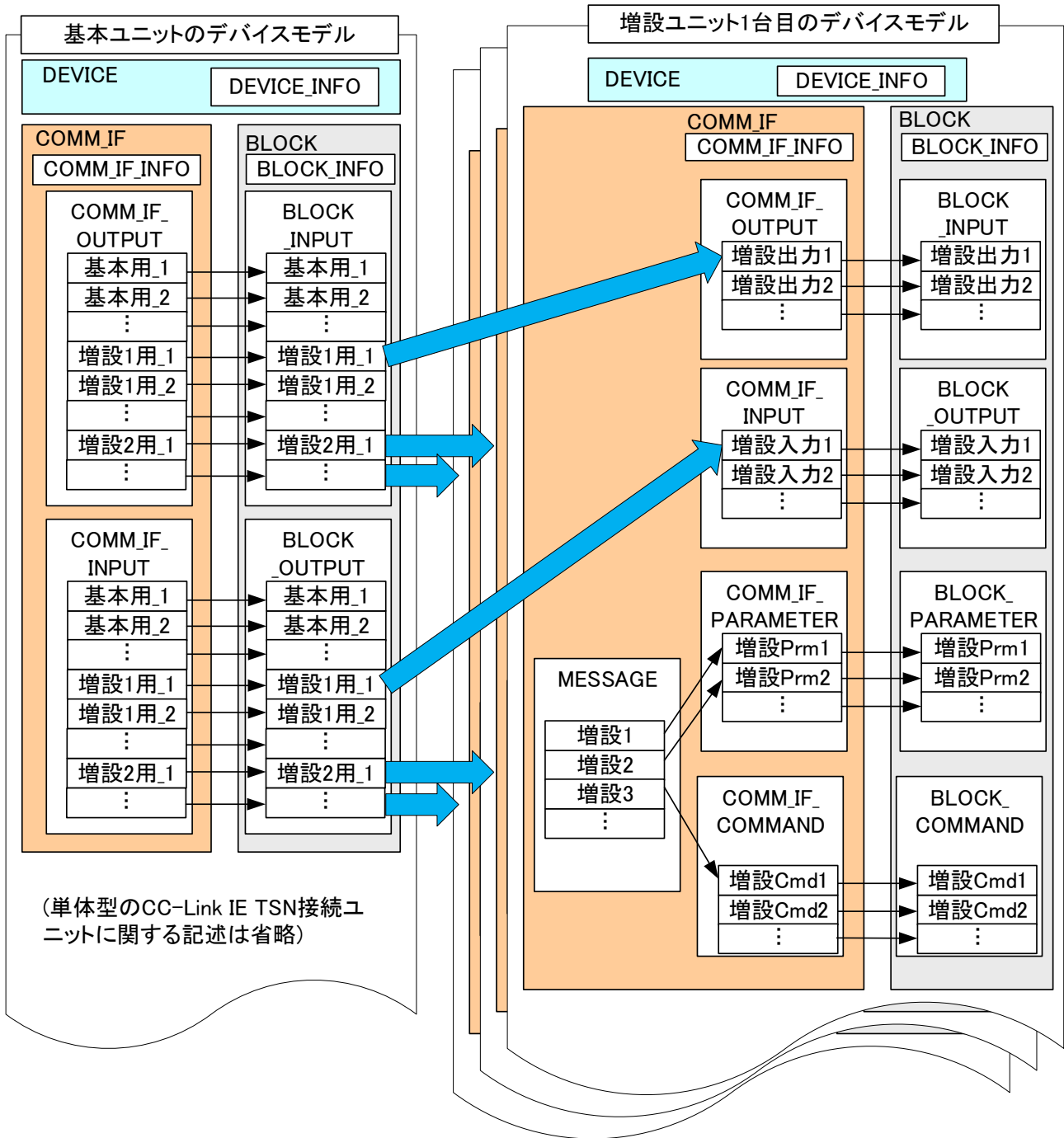
図 4-17 CC-Link IE TSN 基本ユニットと増設ユニットのGSP+ファイルの一般形モデル
