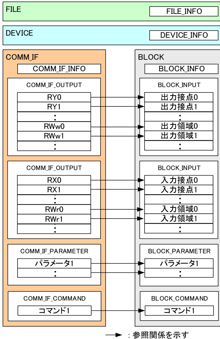
図 4-13 Ethernet接続ユニット用CSP+ファイルの一般形モデル
