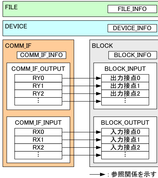
図 4-6 CC-Link リモート I/O 局用 CSP+ファイルのモデル
