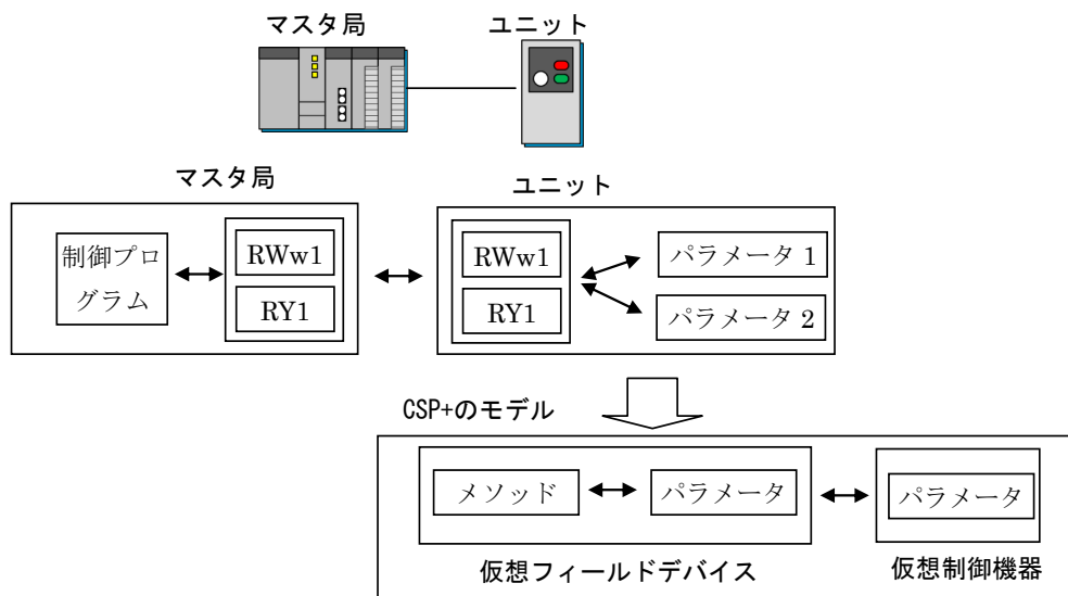
図 3-3 サイクリック伝送によるパラメータ送受信の例
