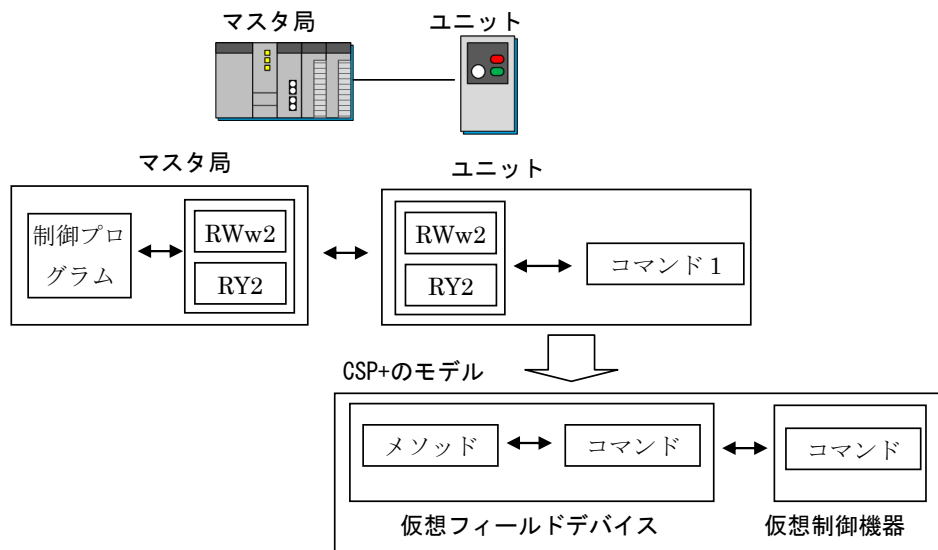
図 3-4 サイクリック伝送によるコマンド送信の例
