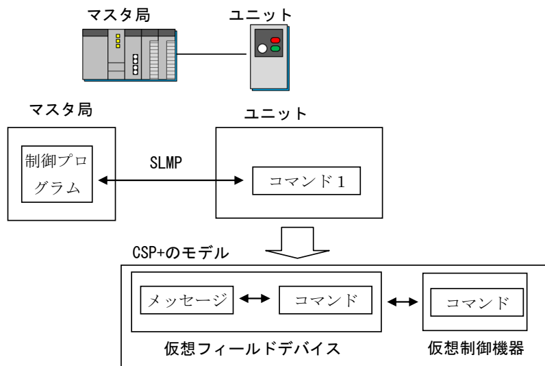
図 3-7 SLMPによるコマンドの送信
