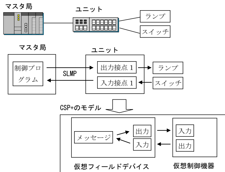
図 3-5 SLMPによる入力・出力
