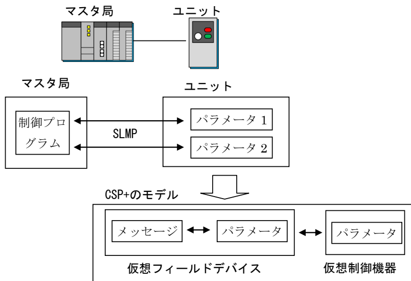
図 3-6 SLMPによるパラメータの送受信
