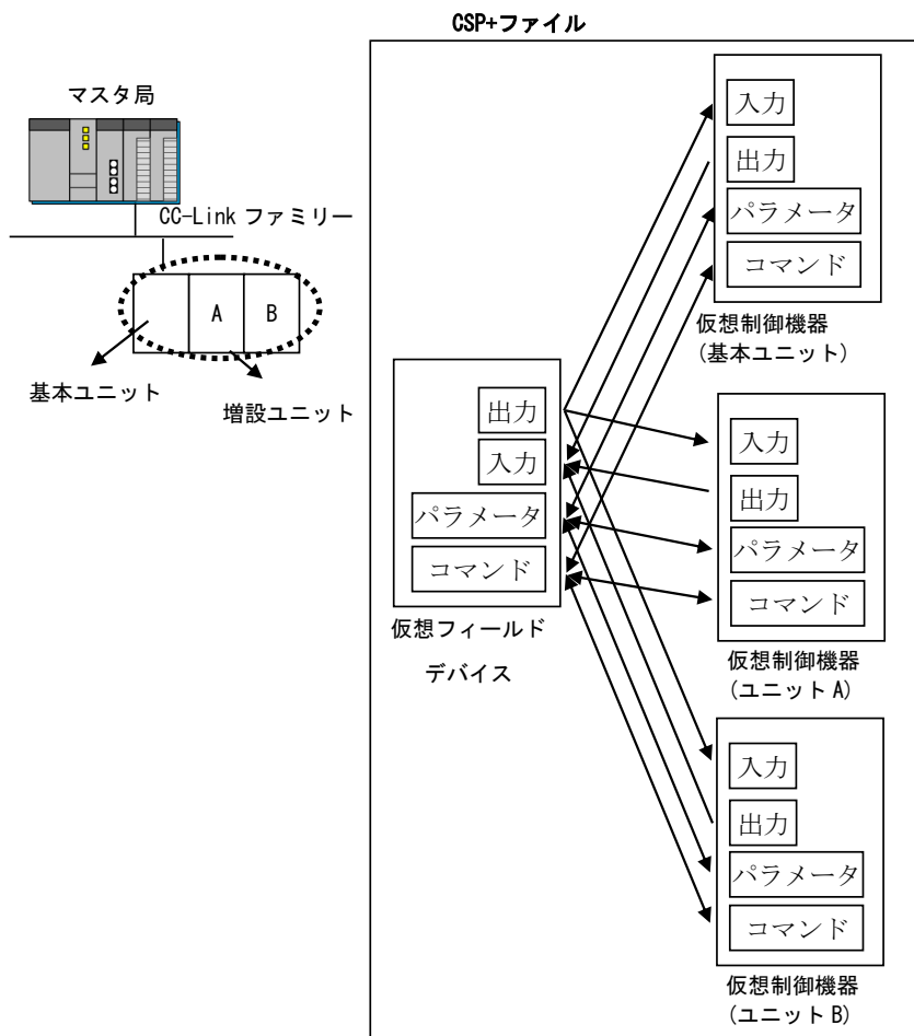
図 3-11 増設ユニットを含む構成で記述する場合のユニットのモデル(基本ユニットと増設ユニットの仮想制御機器を分けて記述する場合)
